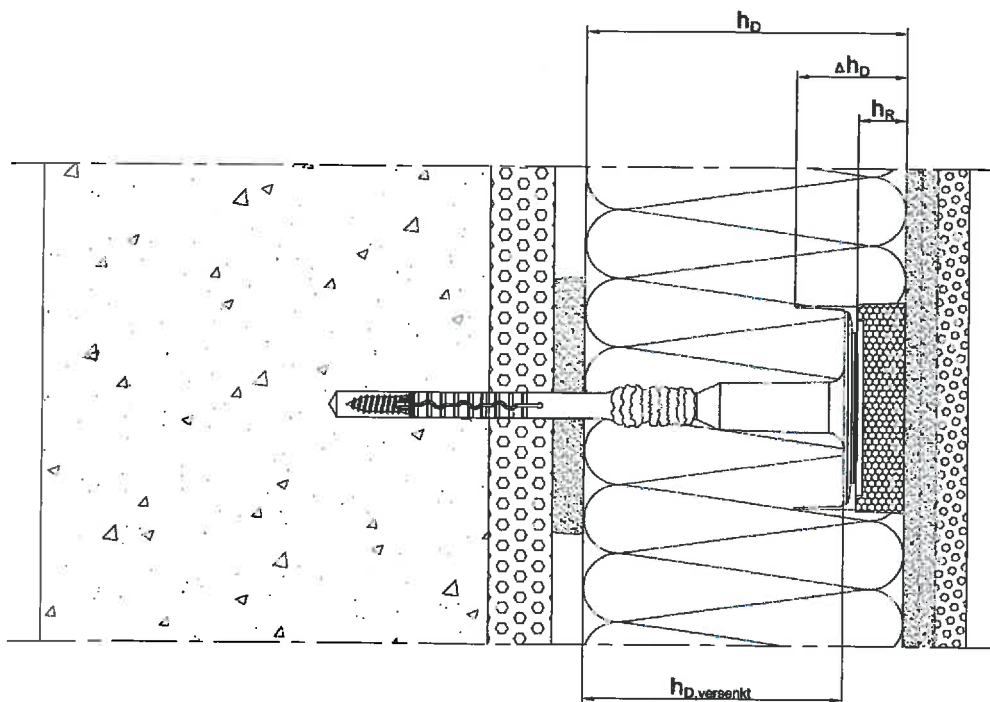
Bild 5.1: ejothem STR U und ejothem STR U 2G (versenkte Montage)
