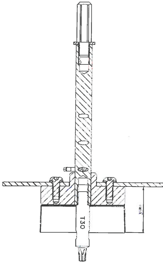
Bild 4.3: ejotherm STR U 2G Montagewerkzeug Typ "L" für Dämmstoffdicken ab 100 mm
