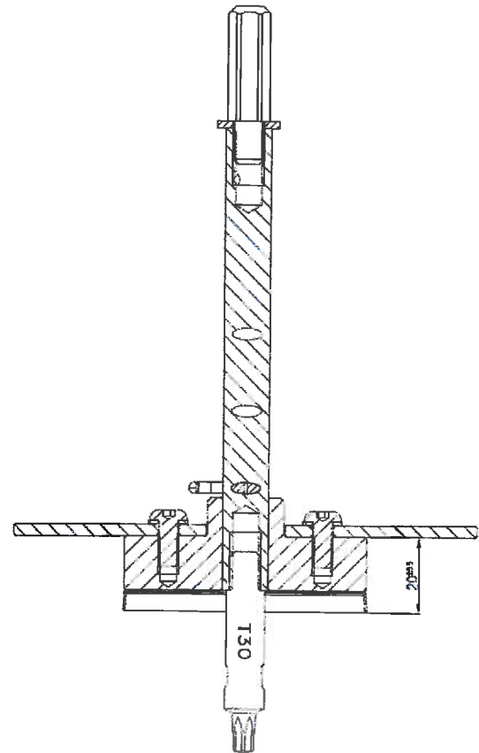
Bild 4.4: ejotherm STR U 2G Montagewerkzeug Typ "S" für Dämmstoffdicken ab 80 mm
